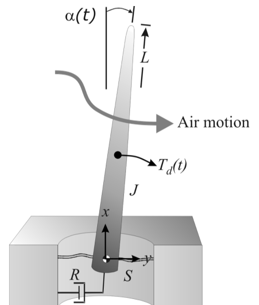
Schematische weergave van een flowgevoelige haarsensor.
